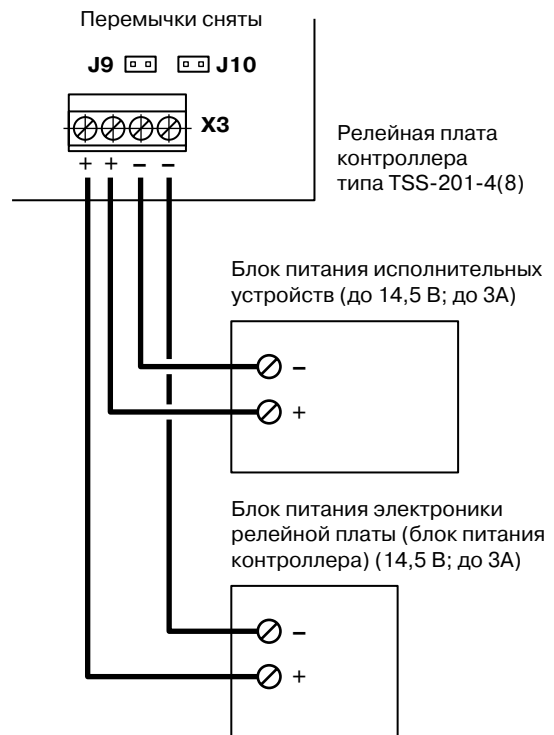
Рис. 10Б Подключение блоков питания к релейной плате при раздельном электропитании исполнительных устройств и электроники платы
