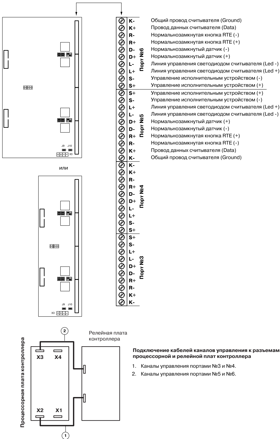
Рис.9 Порты контроллера TSS-201-4Т, служащие для подключения оборудования пунктов прохода
