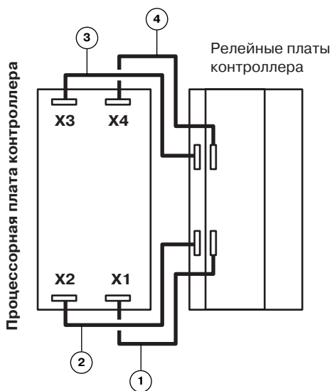
Рис.8 Порты контроллера TSS-201-8Т, служащие для подключения оборудования пунктов прохода
