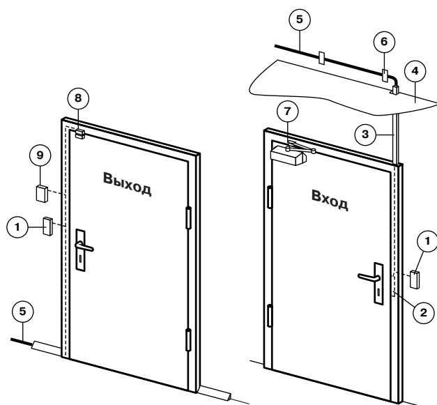
Пример монтажа оборудования двухдверного пункта прохода
