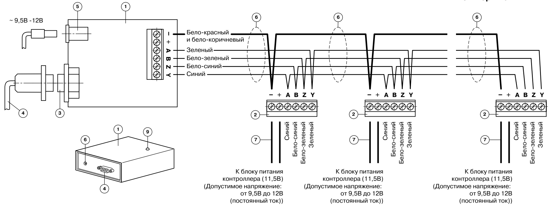
Рис.4 Подключение контроллеров серии TSS-201 к компьютеру мониторинга
