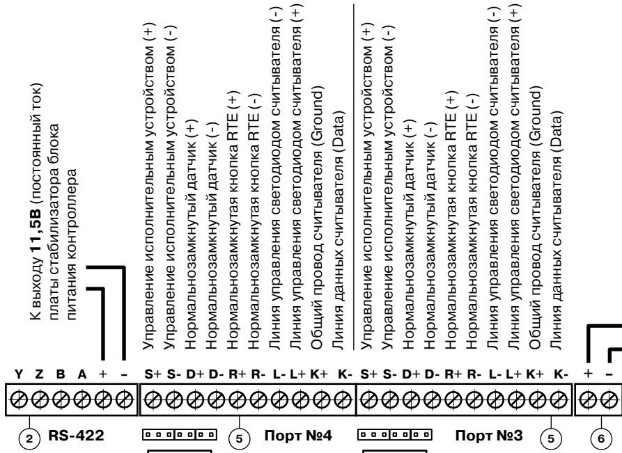
Рис.7 Компоновка и клеммное поле контроллера TSS-201-2T
